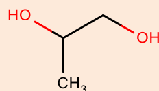
1,2-propanediol CAS: 57-55-6
