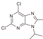
PB02974 CAS: 1313026-86-6
