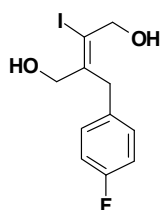
(Z)-2-(4-fluorobenzyl)-3-iodobut-2-ene-1,4-diol
