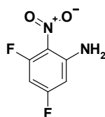
3,5-difluoro-2-nitroaniline
