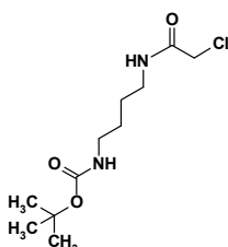
tert-butyl N-[4-(2-chloroacetamido)butyl]carbamate
