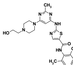
Dasatinib
