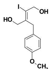
(Z)-2-iodo-3-(4-methoxybenzyl)but-2-ene-1,4-diol
