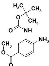
methyl 4-amino-3-[[tert-butoxy]carbonyl]amino]benzoate
