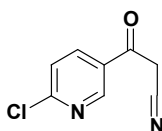
3-(6-chloropyridin-3-yl)-3-oxopropanenitrile
