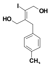
(Z)-2-iodo-3-(4-methylbenzyl)but-2-ene-1,4-diol
