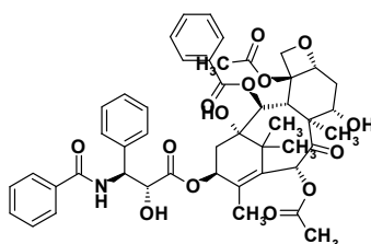
(-)-Paclitaxel; Paclitaxel
