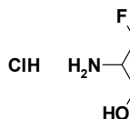
2-amino-3-fluoropropan-1-ol hydrochloride
