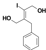
(Z)-2-benzyl-3-iodobut-2-ene-1,4-diol
