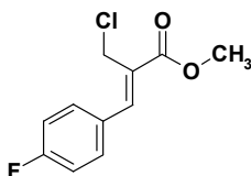
Methyl (Z)-2-(chloromethyl)-3-(4-fluorophenyl)acrylate
