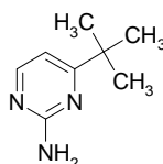
4-tert-butylpyrimidin-2-amine
